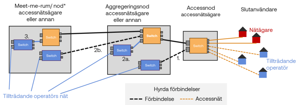
Figur 18 Möjliga tillträdes- och överlämningspunkter för VULA
