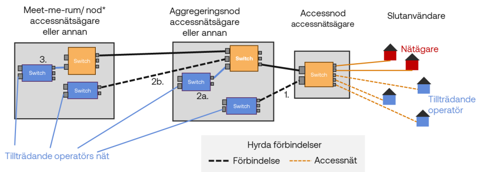
Figur 1 Möjliga tillträdes- och överlämningspunkter för VULA
