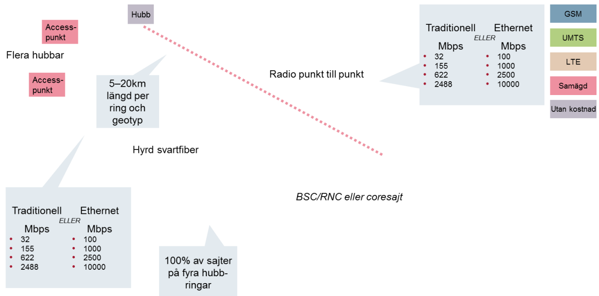
Bild 6.3: Översikt över transmissionen i modellen mellan hubbar och corenätet [Källa: Analys Mason]
