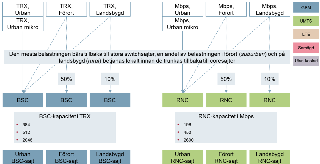
Bild 6.4: Översikt över BSC och RNC i modellen [Källa: Analysys Mason]
