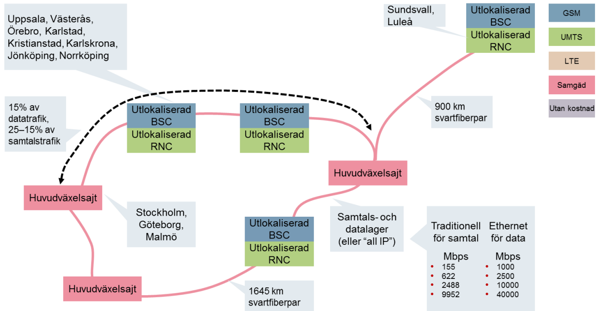
Bild 6.6: Översikt över transmission i corenätet i modellen [Källa: Analysys Mason]
